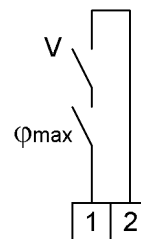
Klemmen 1/2 an der Hauptplatine für Anschluss der Sicherheitskette
