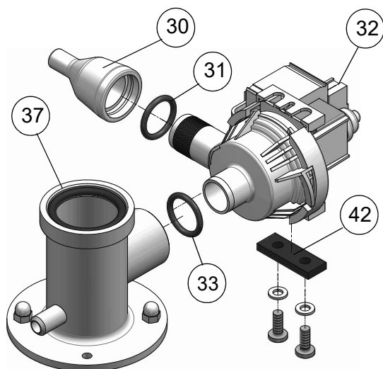
Abschlämppumpe
