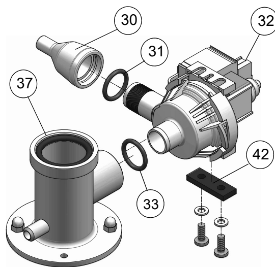
Abschläämpumpe
