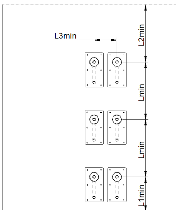
Abb: Abstände der Dampfverteiler
