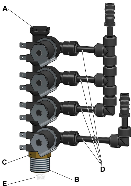
Vierfach-Magnetventil (FLPxx-TPRO)
