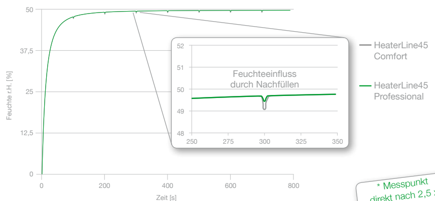
Feuchteverlauf* im Vergleich: HeaterLine Professional gegen HeaterLine Comfort
