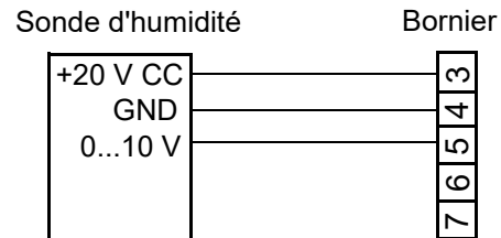
Exemple de raccordement d'une sonde d'humidité 0...10 V
