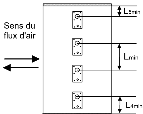
Disposition standard des distributeurs de vapeur:
