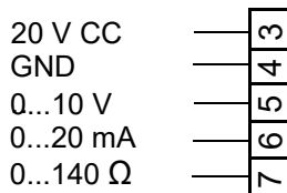
Bornes de connexion pour signaux de commande
